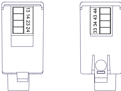
Disposizione morsetti Terminal blocks position
